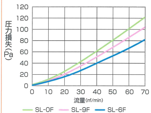
流量と圧力損失
